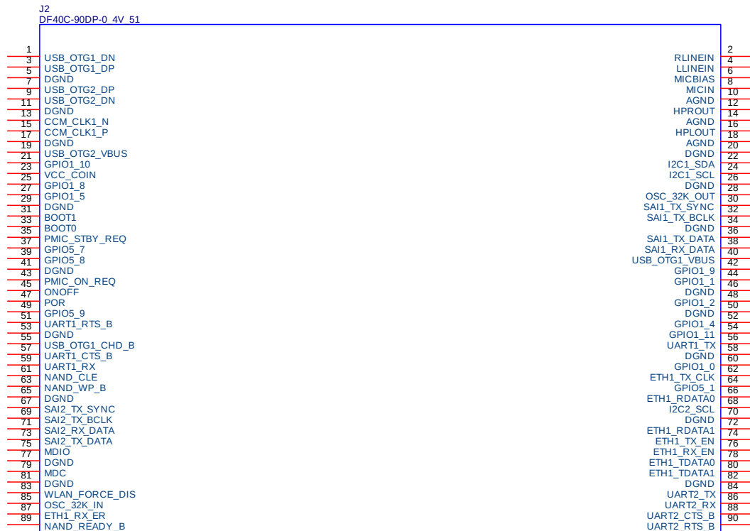
Figure 3-2 SOM J2 Connector
