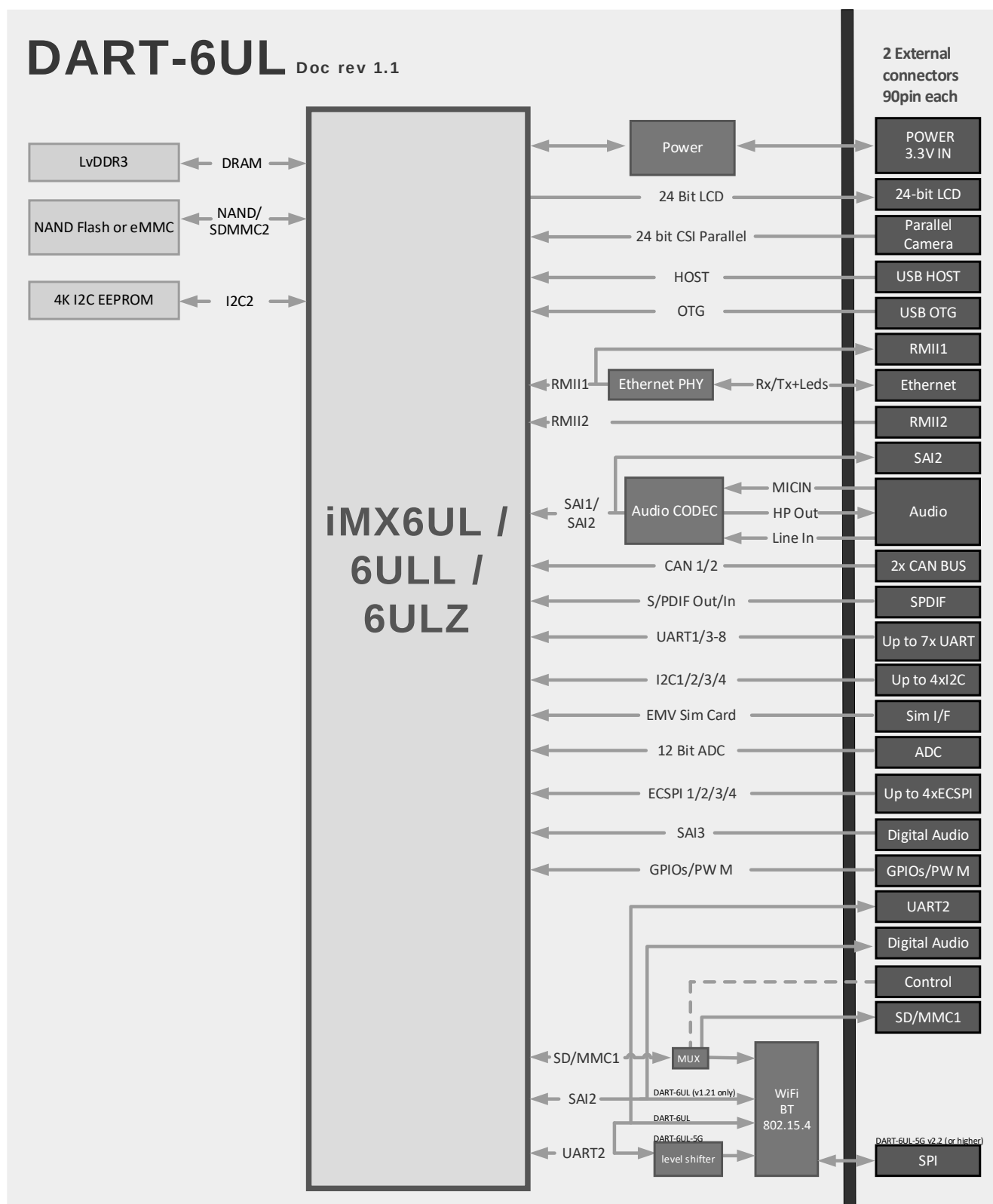
Figure 1-1 SOM Block Diagram
